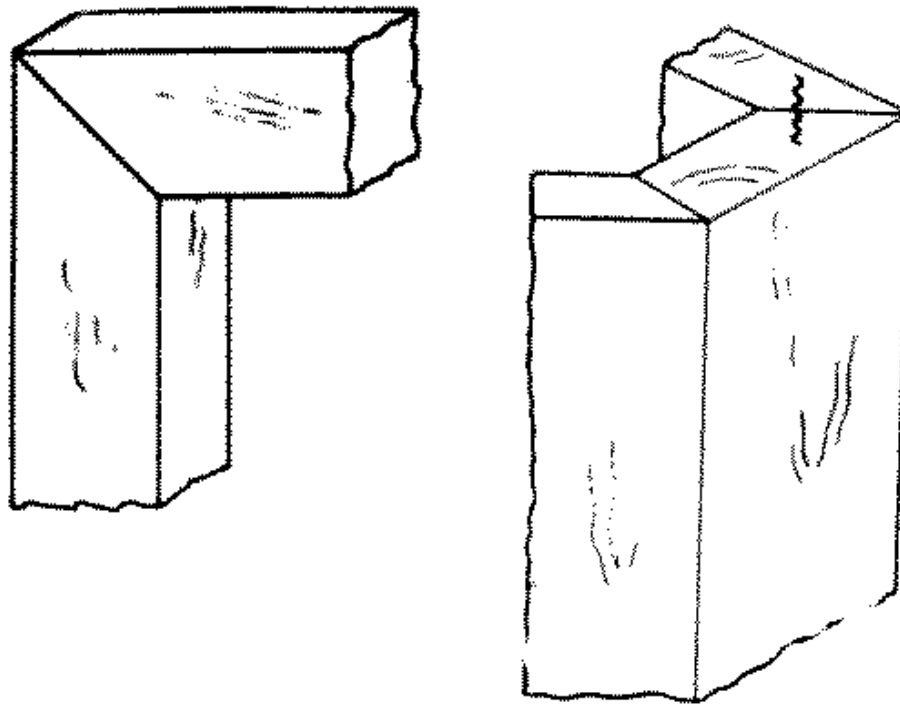
Fig. 268-52 Miter
