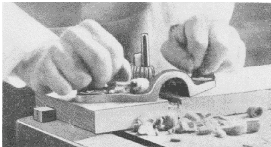
Fig. 122. Using a Router-Plane.
