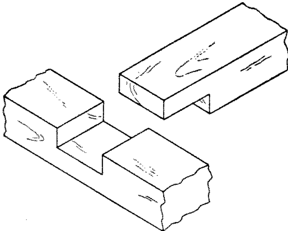
Fig. 265-15 Middle lap
