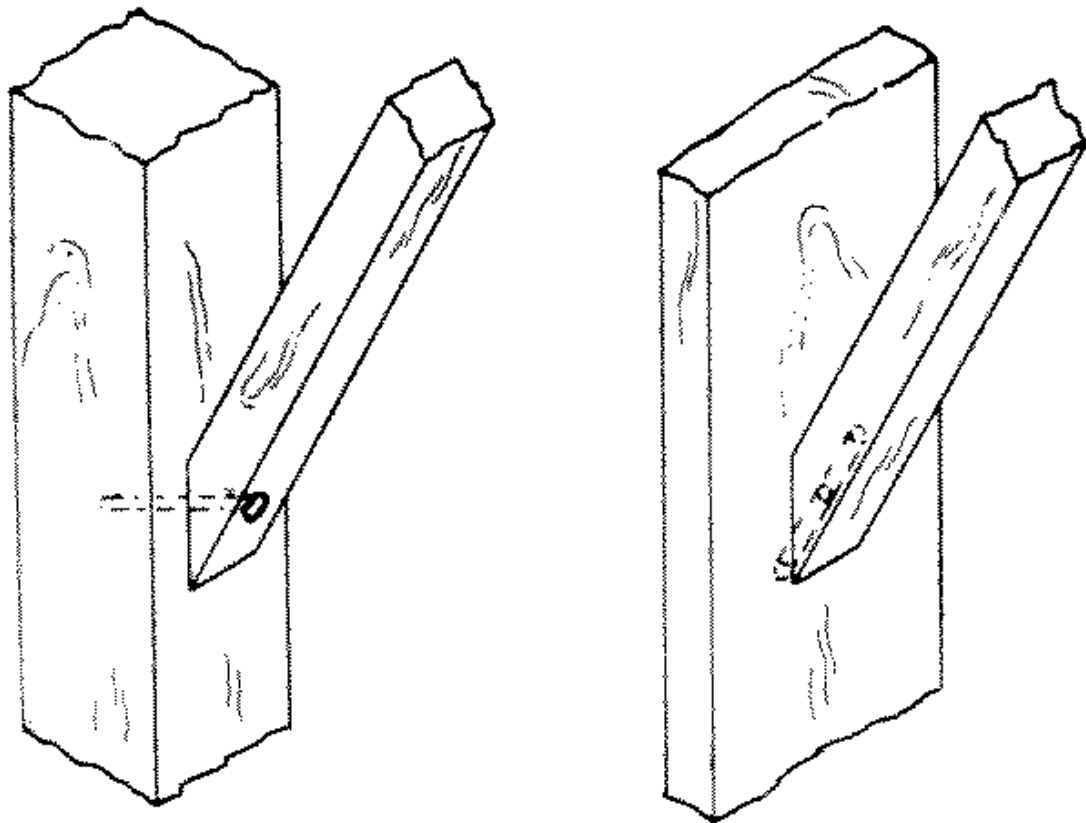
Fig. 269-65 Brace
