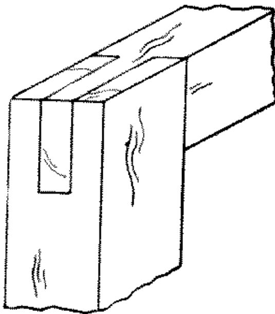
Fig. 267-46 Slip
