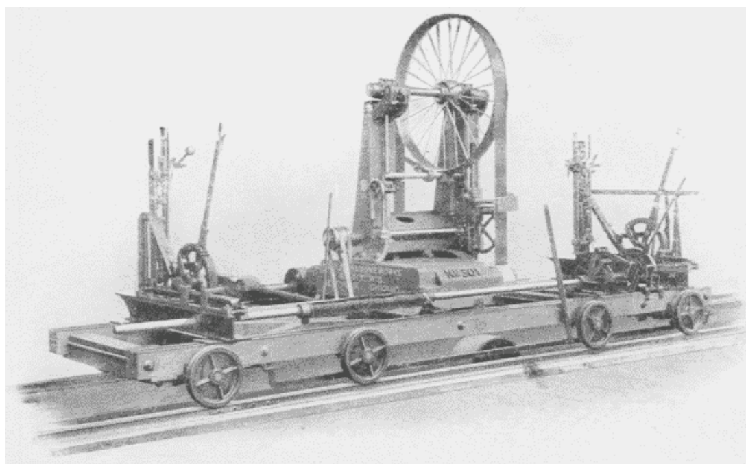
Fig. 34. Band-Saw.
