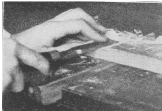
Fig. 71. Chiseling Out a Dado. (Second Step).
