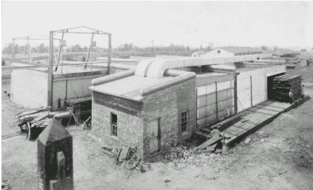
Fig. 57. Lumber-Kiln.
