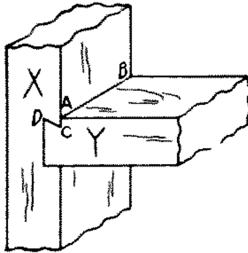
Fig. 266-28 Dovetail dado
