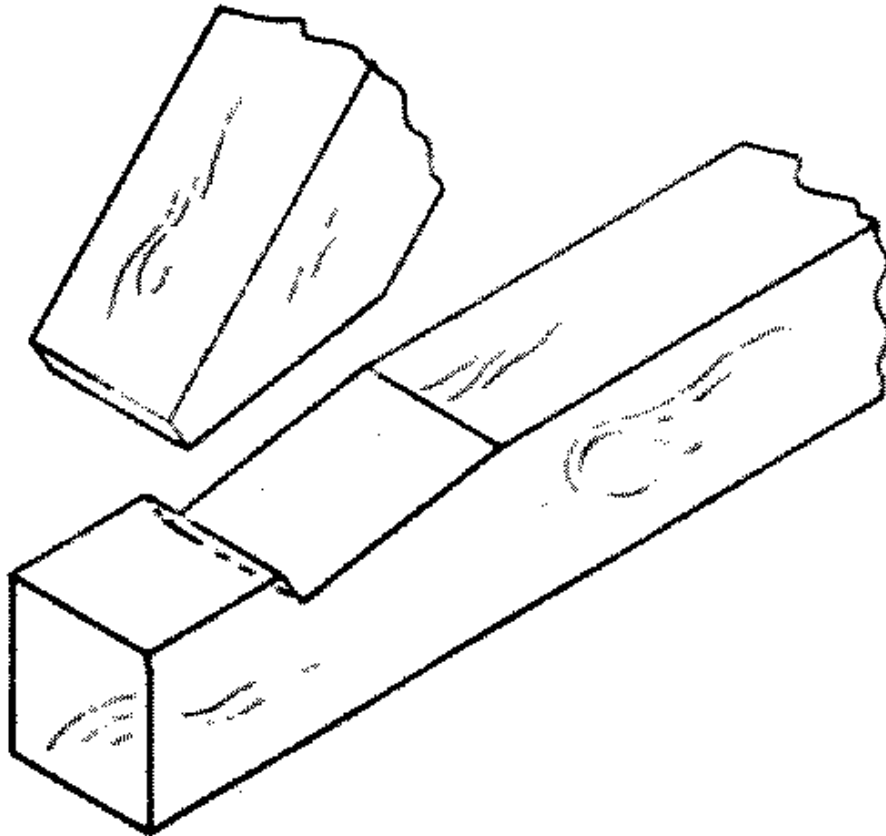
Fig. 268-64 Oblique thrust
