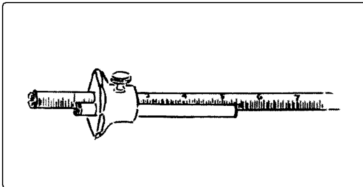
Fig. 217. Roller Mortise-Gage.
