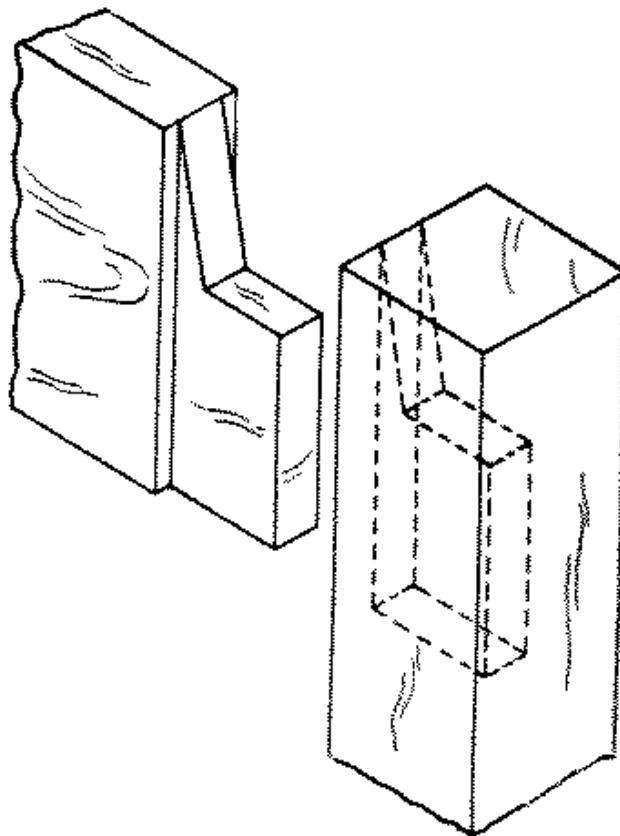
Fig. 267-43 Table haunching
