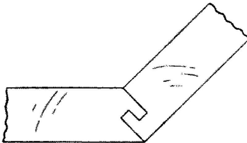
Fig. 268-60 Double tongue miter
