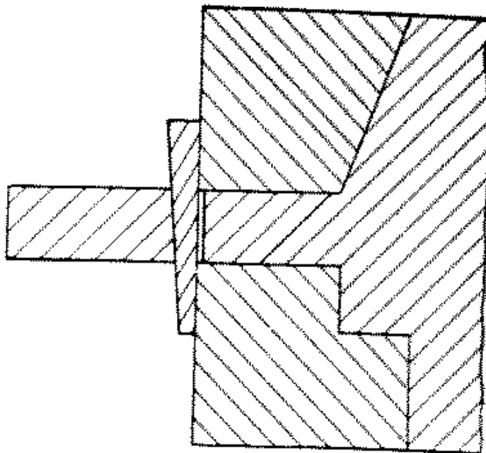
Fig. 267-40 Tusk tenon
