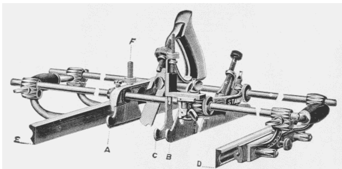
Fig. 117. Universal Plane.
