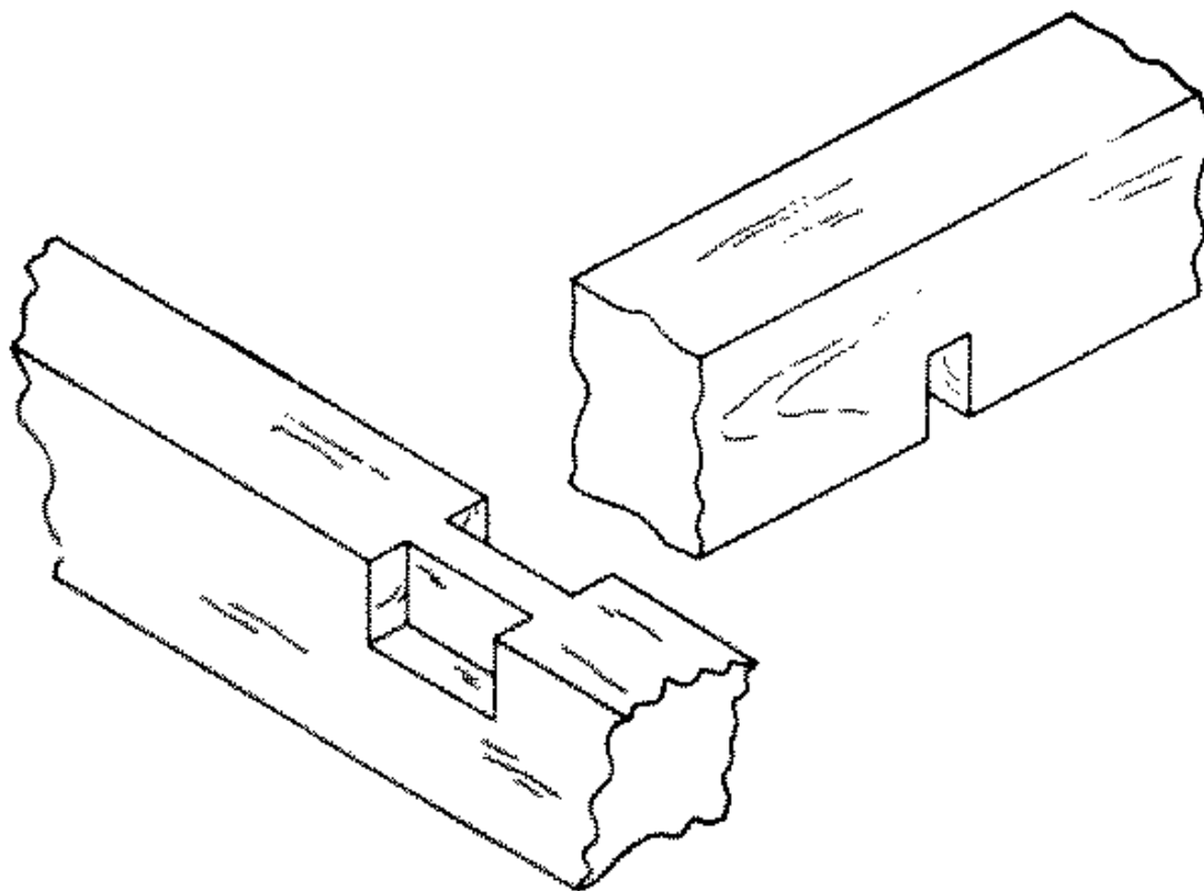
Fig. 265-22 Cogged
