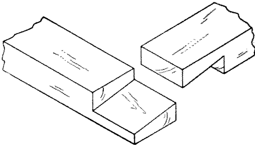
Fig. 265-19 Beveled halving
