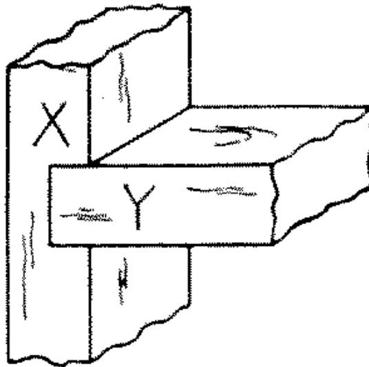
Fig. 266-25 Dado
