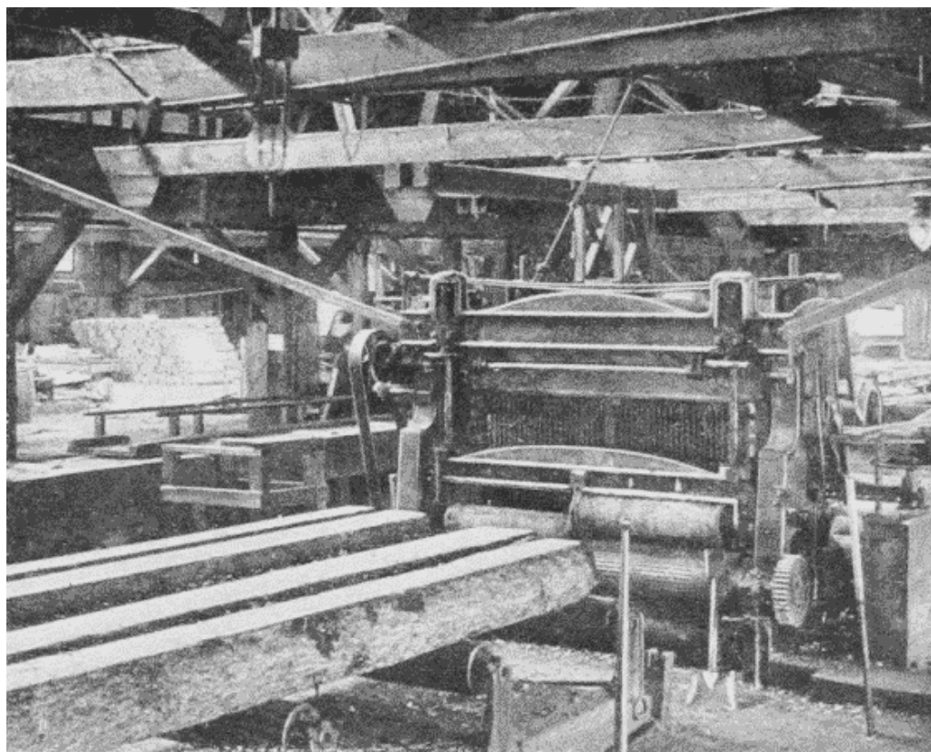
Fig. 33. Gang-Saw.
