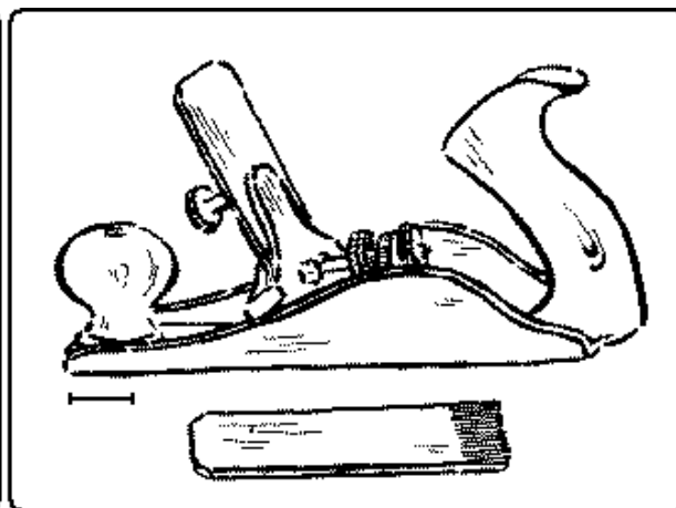
Fig. 111. Scratch-Plane and Scraper-Plane.
