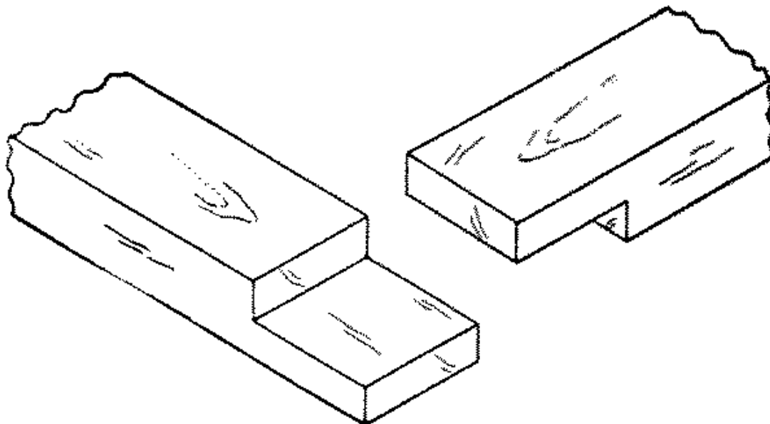
Fig. 265-16 End lap
